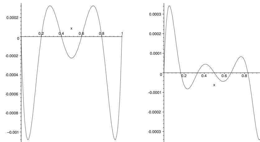
Figura: Representació gràfica de \omega(x) = (x - x_0) \dots (x - x_n) amb abscisses equiespaiades a [0, 1] ( x_i = i/n , i = 0 \div n ), per n = 5 (esquerra) i n = 6 (dreta).
