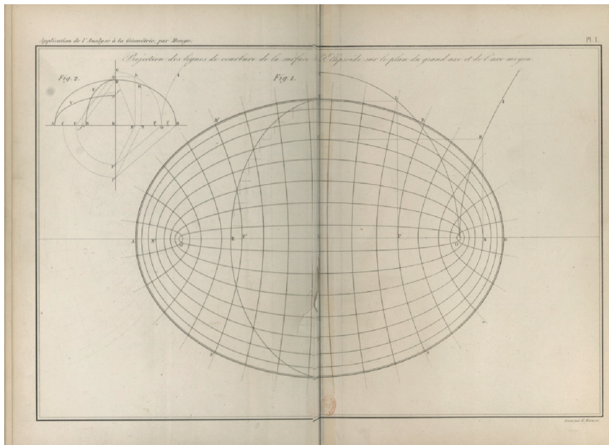
FIGURA 10: Línies de curvatura de l'el·lipsoide [M18].
