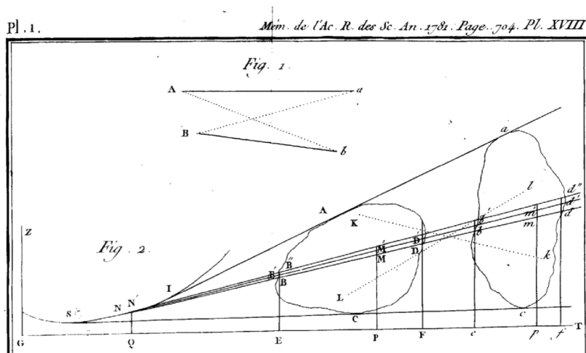
FIGURA 5: Dibuix de Monge del déblai i el remblai . Les rectes determinen una àrea igual sobre cada figura, ABD = abd . Són tangents a una corba. BD ha d'anar a bd .
