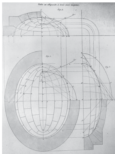
FIGURA 11: Dovelles sobre el·lipsoide.
