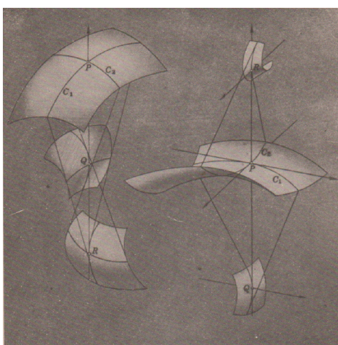
FIGURA 8: Dibuix de Struik [T15, p. 108]. 29
