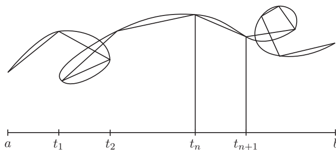
Aproximació poligonal. 10
