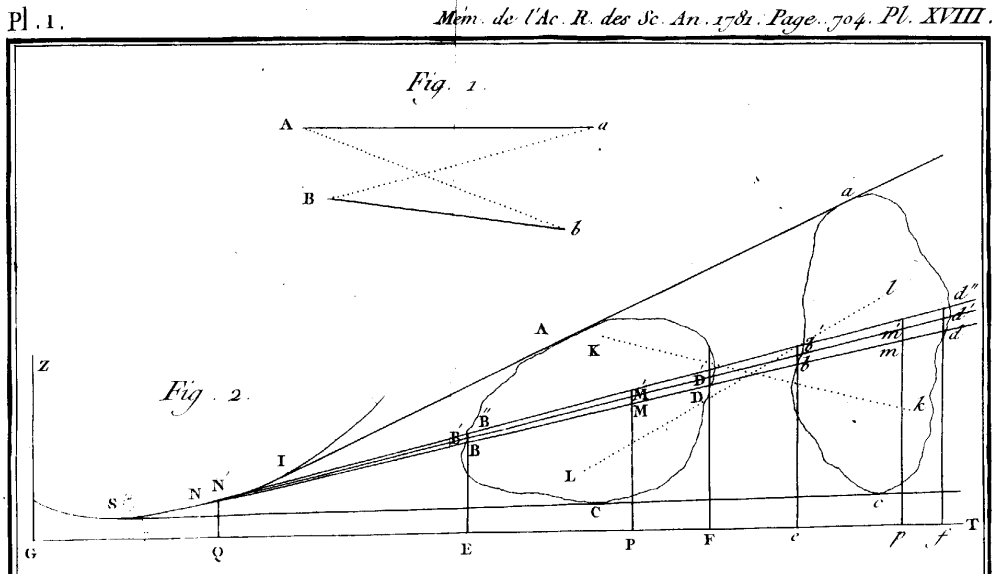
Figura 7. Dibuix de Monge del ‘déblai’ i el ‘remblai’. Les rectes determinen igual àrea sobre cada figura, ABD = abd . Són tangents a una corba. BD ha d’anar a bd .
