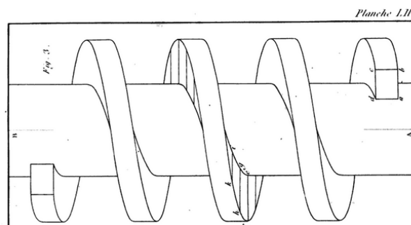
Vis à filet quarré. Detall de la planxa LII de Vallée, [A521].
