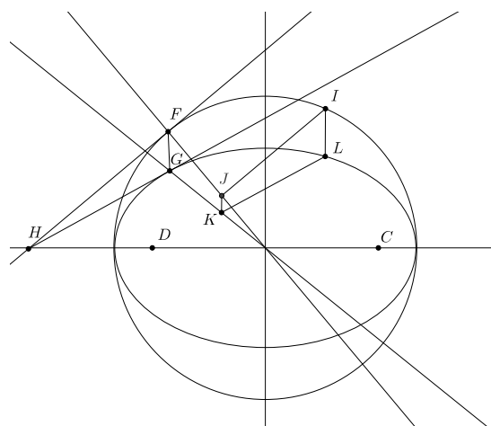
Figura 2.7: El·lipse i circumferència.
