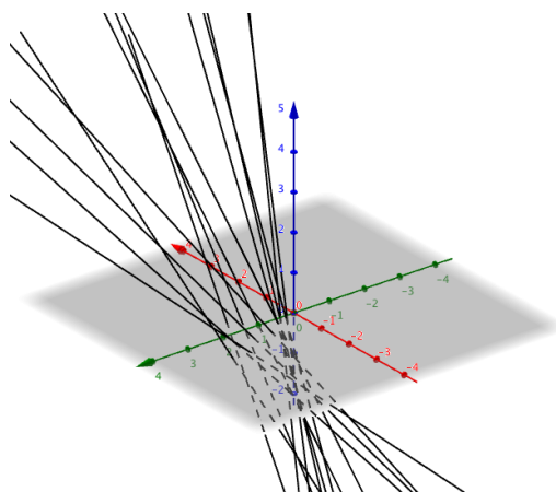
Figura 11. La foliació donada pels plans ortogonals a aquestes rectes no és integrable.
