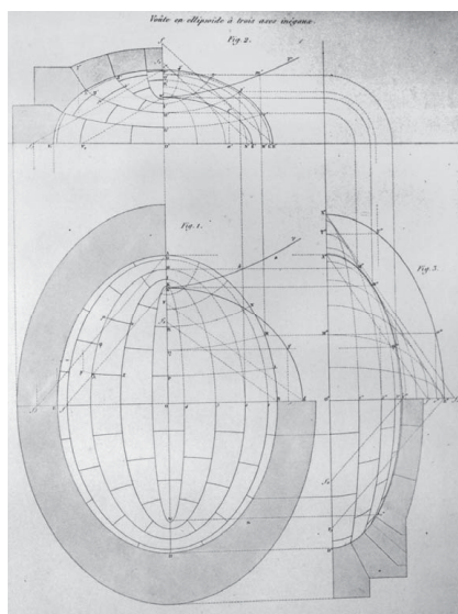
Figura 13. Dovelles sobre el·lipsoïde.
