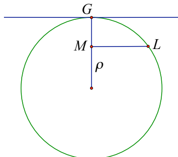
Figura 2.8: Radi de curvatura.
