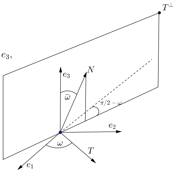
Figura 9.18: Trièdres de Darboux i Frenet.
