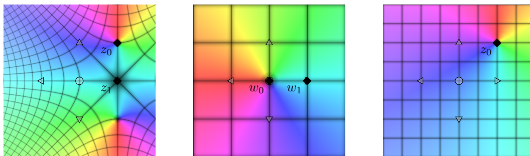
Figura 3.2.: En la imatge central, trobem la graella en el pla complex en 2Q . La primera representa f(z) = z^2 - 2z + 2 en el mateix domini amb un gràfic de colors en coordenades cartesianes (vegeu la secció 2.1). Recordem que es representa la preimatge de la graella per la funció f . Prenem z_0 = 1 + i , w_0 = f(z_0) = 0 i f'(z_0) = 2i . La tercera imatge és l'aproximació lineal w_0 + f'(z_0)(z - z_0) , que envia z_0 a w_0 i produeix una rotació de \frac{\pi}{2} i una dilatació de raó 2 entorn de z_0 . En general, veiem que els angles de la graella es preserven llevat del punt z_1 = 1 + 0i , on s'anul·la la derivada, i l'aproximació (en aquest cas igualtat) és de grau 2: w = f(z_1) + \frac{f''(z_1)}{2}(z - z_1)^2 .
