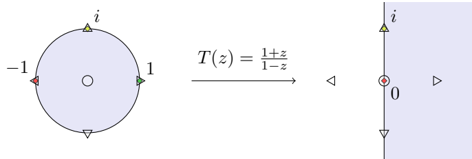
Figura 7.8.: L'homografia T(z) = \frac{1+z}{1-z} envia el disc unitat al semiplà de la dreta.
