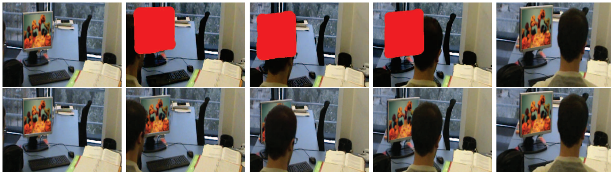
Figura 2: Alteració d'un objecte en un vídeo. En aquest exemple l'usuari modifica la imatge sobre el monitor de l'ordinador en el primer i últim fotograma i marca una regió d'edició. L'objectiu de l'algorisme és doncs propagar la modificació als dels fotogrames restants en la regió d'edició.
