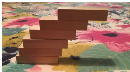
Figura 1. Torre de sis peces construïda basant-se en la sèrie harmònica, veure la Secció 4.10.
