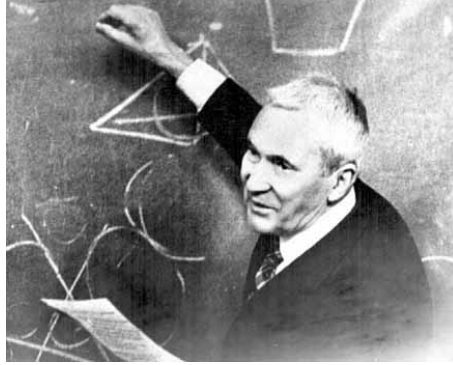
Figura 10. A. N. Kolmogórov
