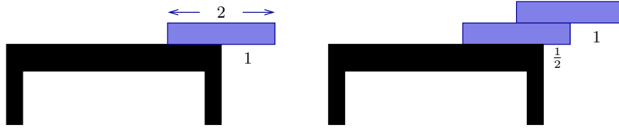
Figura 7. Torres amb una o dues peces.
