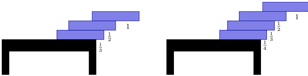
Figura 8. Torres amb tres o quatre peces.
