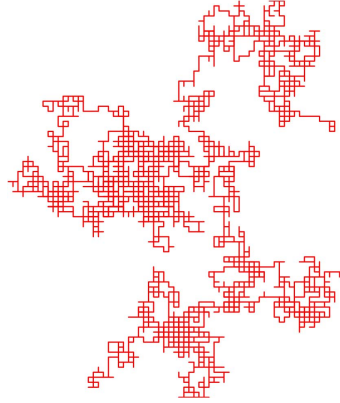
Figura 5. Passeig aleatori al pla.
