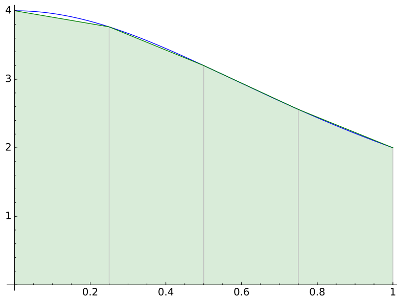
Figura 5. Fórmula dels trapezis per a n = 4 .
