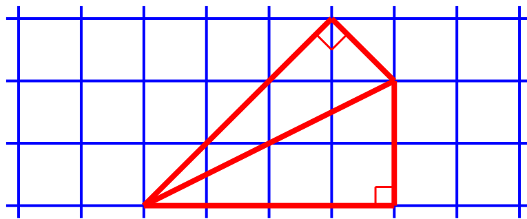
Figura 6. Suma d'arctangents
