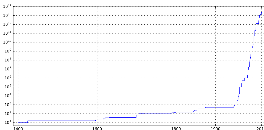
Figura 1. Rècords de computació dels dígitos de \pi . Font: Wikipedia, abril 2018
