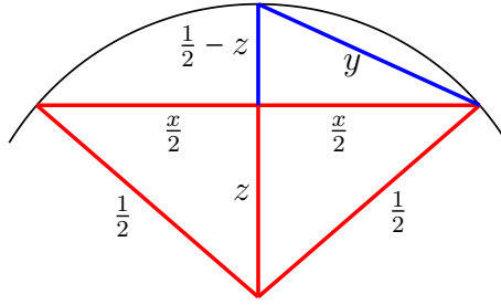
Figura 4. Càlcul dels costats del polígon
