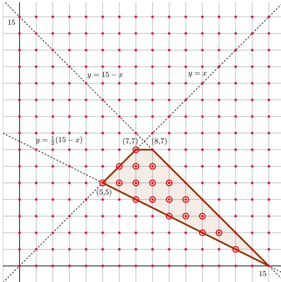
Figura 2: El conjunto \mathcal{P}(15) .
