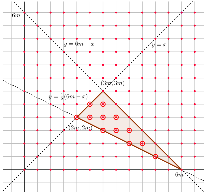
Figura 7: \mathcal{P}(n) para n = 6m .
