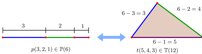
Figura 6: Relación P(n) = T(2n) , con n = 6 .
