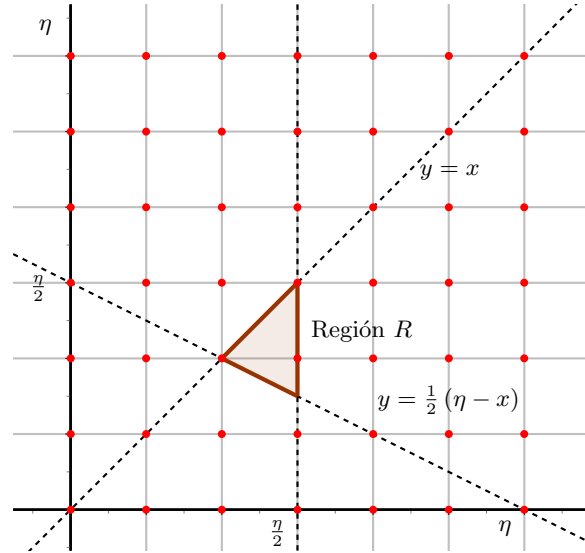
Figura 3: La Región R .
