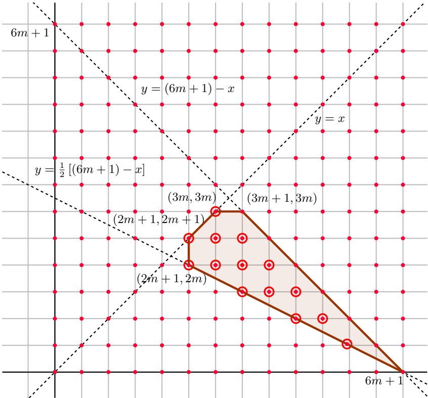
Figura 8: \mathcal{P}(n) para n = 6m + 1 .
