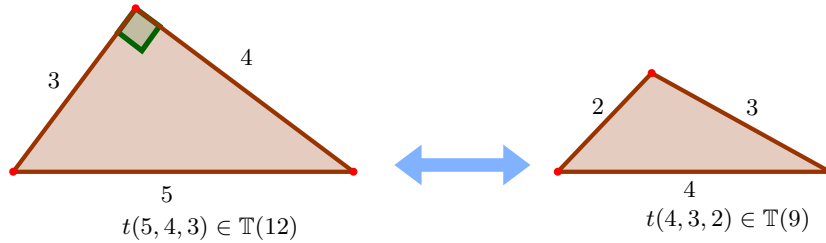
Figura 5: Relación T(2n) = T(2n - 3) , con n = 6 .
