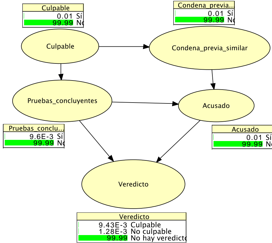
Figura 2: Probabilidades marginales.
