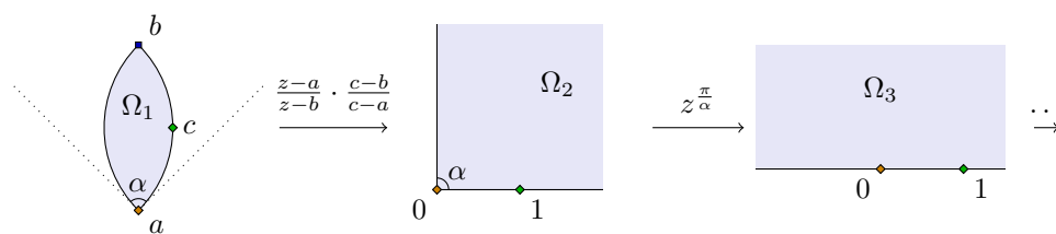
Figura 7.18: Aplicació de Riemann d'una lent (serveix també per segments circulars i lúnules).
