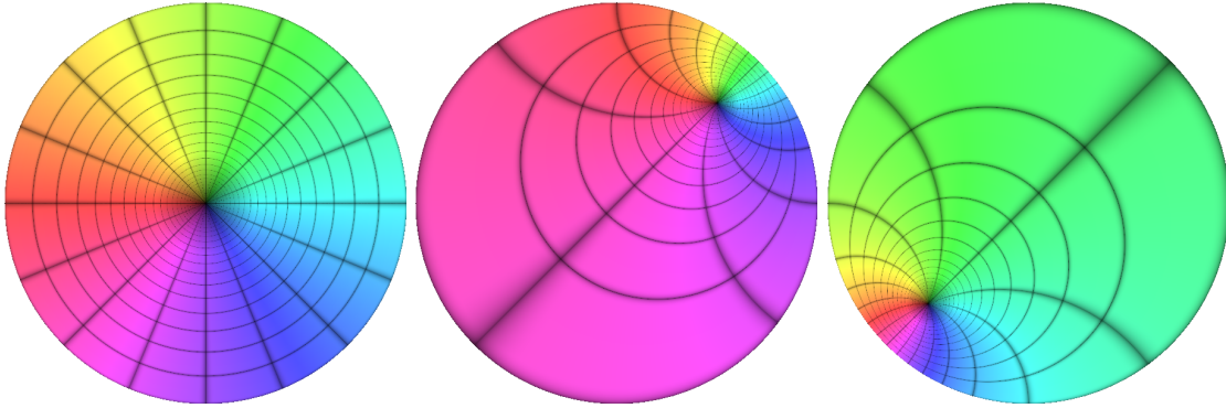
Figura 7.11: Automorfisme identitat del disc unitat representats en polars (inclou radis d'angle k\pi/8 ), automorfisme del disc T(z) = \frac{z-a}{1-\bar{a}z} amb a = \frac{1}{2} + \frac{i}{2} i automorfisme invers.
