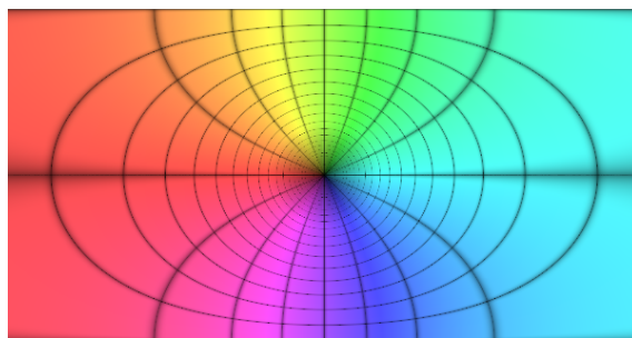
Figura 7.17: Aplicació de Riemann de la banda \Omega_1 , coloració de la figura 7.11.
