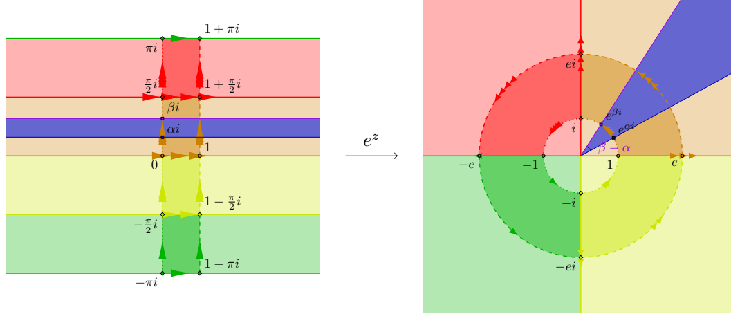
Figura 7.15: Acció de la funció exponencial en bandes horitzontals i en rectangles paral·lels als eixos. Bandes horitzontals d'amplada \gamma van a sectors d'obertura \gamma .
