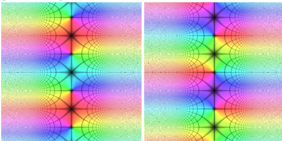
Figura 3.3: Cosinus hiperbòlic i sinus hiperbòlic.
