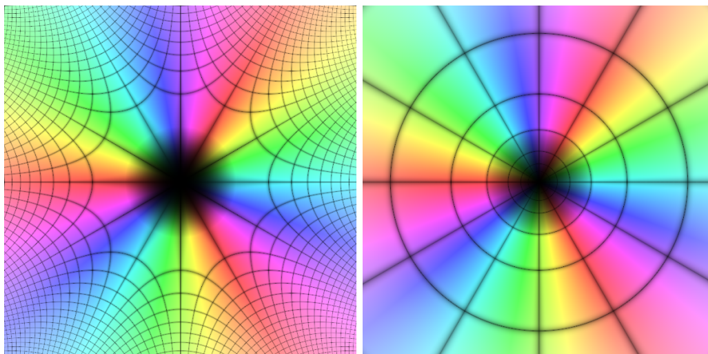
Figura 2.4: Representem el polinomi z^3 entre -2 - 2i i 2 + 2i . Notem que si w \neq 0 , aleshores té tres arrels cúbiques, que són els vèrtexs d'un triangle equilàter centrat a l'origen.
