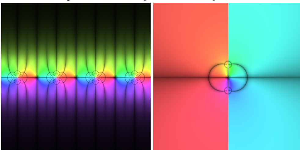
Figura 3.4: Tangent i branca principal de l'arctangent, vegeu l'exercici 3.5.5.
