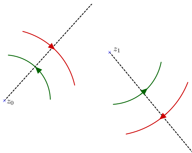
Figura 5.2: Podem observar els camins verds que intersequen en sentit positiu o antihorari i els vermells en negatiu o horari.
