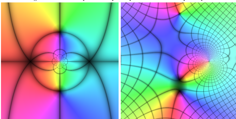
Figura 3.6: \frac{1}{2} \left( z + \frac{1}{z} \right) i \frac{z^3+2z+i}{z-1} , de -2-2i a 2+2i , presenten singularitats, vegeu l'exercici 2.1.7.
