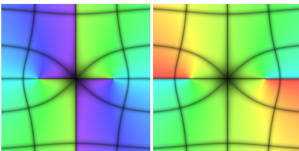
Figura 3.7: Determinació principal de \sqrt{z^2 - 1} i de i\sqrt{1 - z^2} , vegeu l'exercici 2.5.3.
