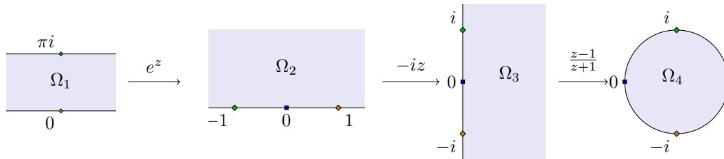
Figura 7.16: Aplicació de Riemann de la banda horitzontal.
