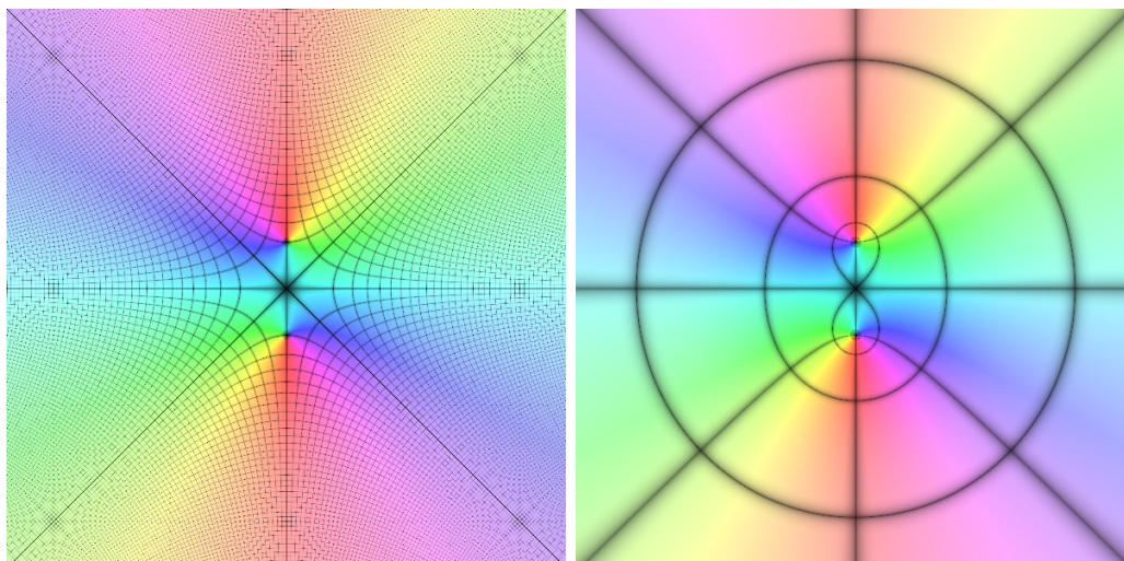
Figura 2.2: Dibuixem la funció f(z) = z^2 + 1 en el mateix domini que abans (des de -6 - 6i fins a 6 + 6i ). Notem que a \pm i , la funció val zero. A l'esquerra la graella correspon als punts d'imatge amb una coordenada entera (corbes de nivell de les parts real i imaginària), a la dreta als d'imatge en els eixos o bé en els cercles de radi e^k (corbes de nivell de mòdul i argument), vegeu figura 2.1.
