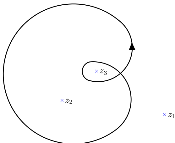
Figura 5.1: Tenim \text{Ind}(\gamma, z_1) = 0 , ja que des de z_1 podem observar tot el camí sense haver de “girar” sobre nosaltres mateixos. En canvi, \text{Ind}(\gamma, z_2) = 1 perquè ens cal fer una volta, i \text{Ind}(\gamma, z_3) = 2 perquè ens cal fer dues voltes per resseguir el camí amb la mirada si ens situem en cada un d’aquests punts.
