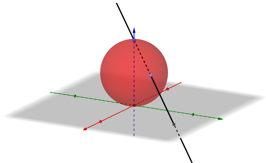
Figura 7.2: La projecció estereogràfica.
