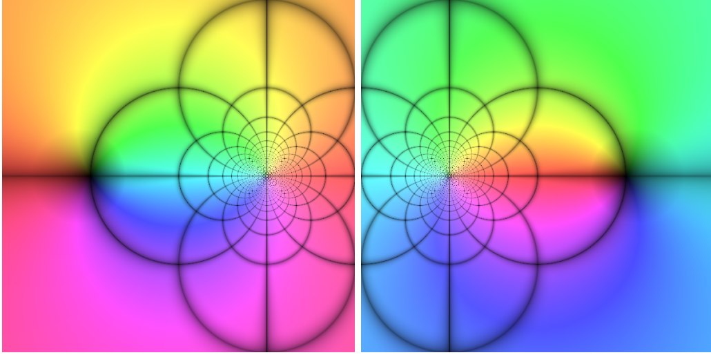
Figura 7.8: L'homografia T(z) = \frac{1+z}{1-z} i la seva inversa, vegeu l'exemple 7.17. Notem que T té pol simple en z = 1 i zero simple en z = -1 , i que les corbes de nivell són circumferències generalitzades que passen pel pol.
