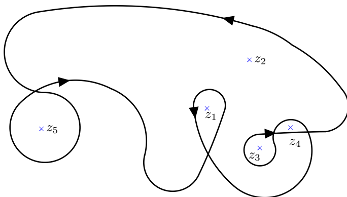
Figura 5.3: Per a calcular l'índex de \gamma respecte a z_j , tracem una semirecta partint del punt i sumem interseccions amb la corba en sentit positiu i restem les de sentit negatiu, tal com il·lustra la figura 5.2.
