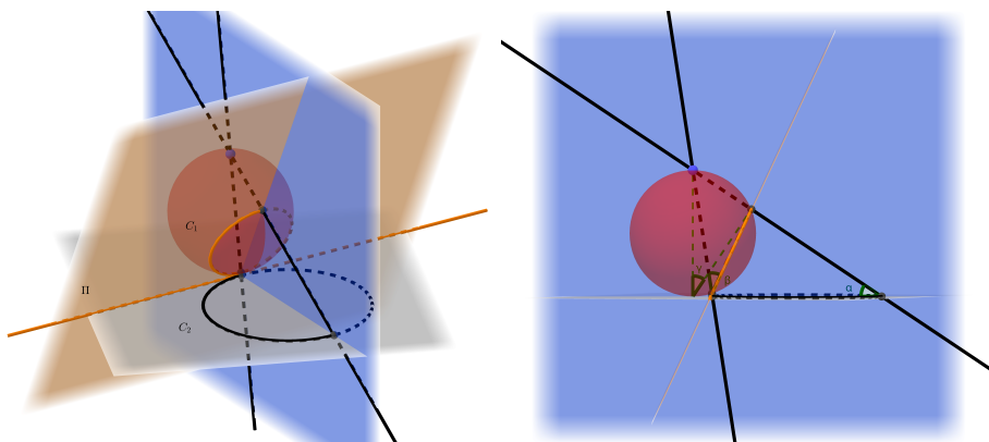
Figura 7.4: La projecció estereogràfica envia circumferències que no passen pel pol nord a circumferències.
