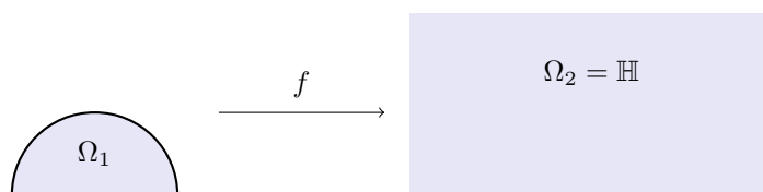
Figura 7.13: Volem trobar una representació f : \Omega_1 \rightarrow \mathbb{H} .
