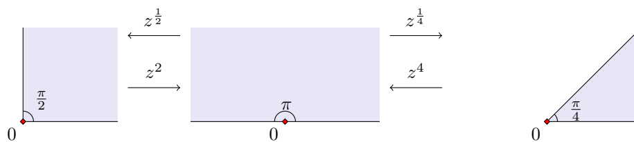
Figura 7.12: Acció de les potències en sectors.
