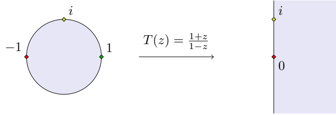
Figura 7.9: L'homografia T(z) = \frac{1+z}{1-z} envia el disc unitat al semiplà de la dreta.
