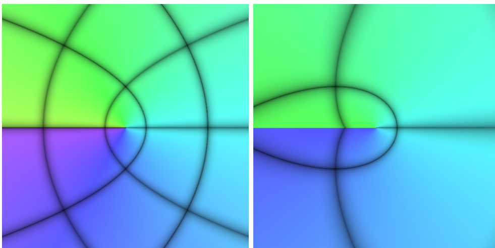
Figura 3.5: Arrel quadrada principal i arrel cúbica principal.
