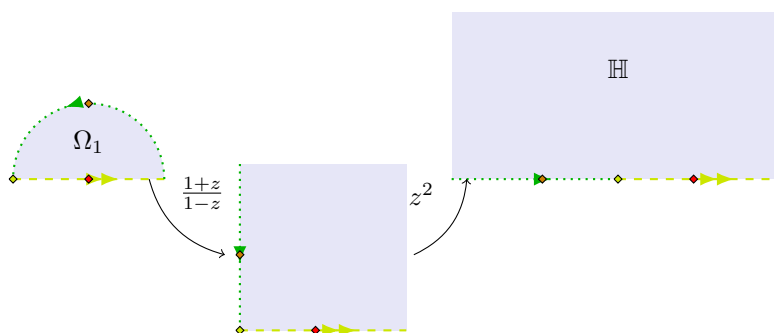
Figura 7.14: Representació f : \Omega_1 \rightarrow \mathbb{H} obtinguda per composició.
